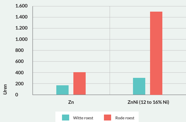
Vergelijking van ZnNi en Zn-coatings op corrosiebestendigheid (Neutrale zoutproei (ASTM B117))
